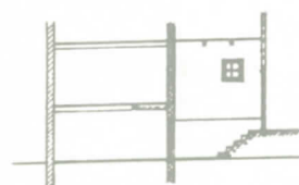
DOORSNED Kelder
