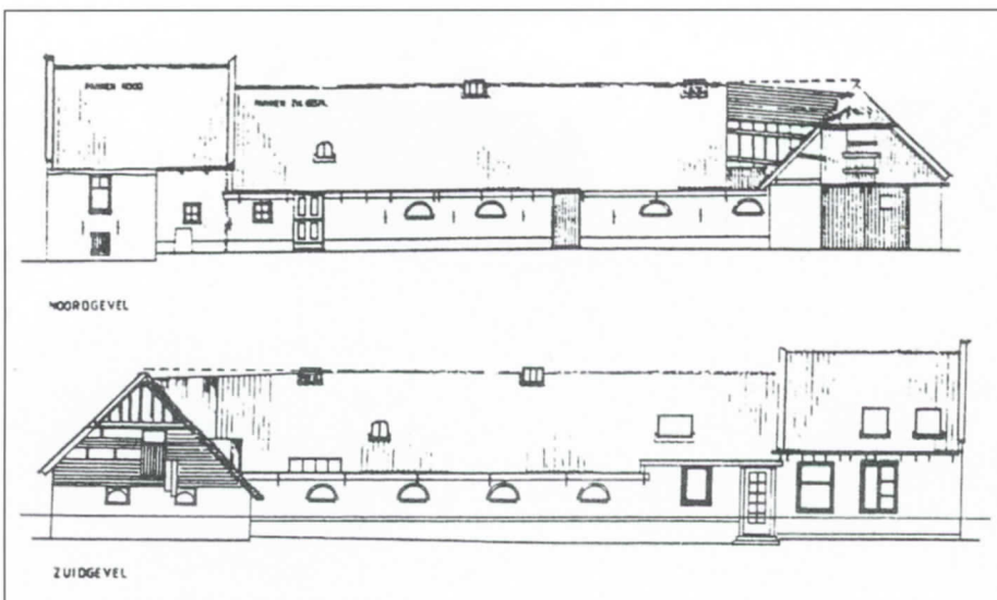
Maattekening van boerderij 'Zeldenrust'
