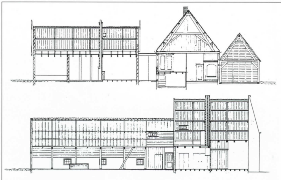
Maattekening van boerderij 'Vredehof'
