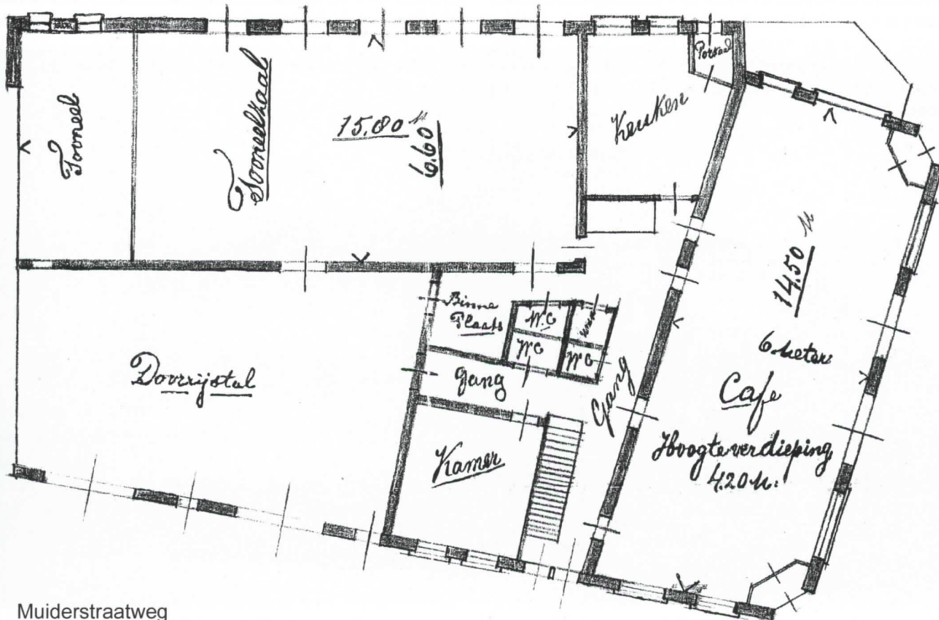
Grondplan van het nieuw te bouwen "Café De Reiger" met café, keuken, vergaderkamer, grote toneelzaal en doorrijstal (coll. Gemeentearchief Diemen).
