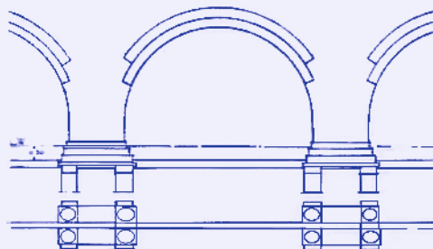
06.08 Een houten paalfundering met een spaarbogenconstructie is meestal onzichtbaar omdat die onder de grond zit.
